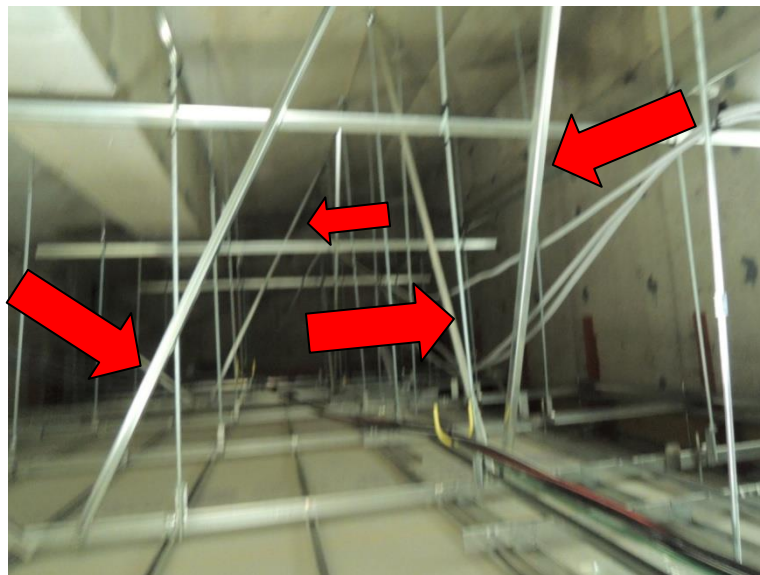
○吊り天井の補強……斜めに支持材を入れて補強
