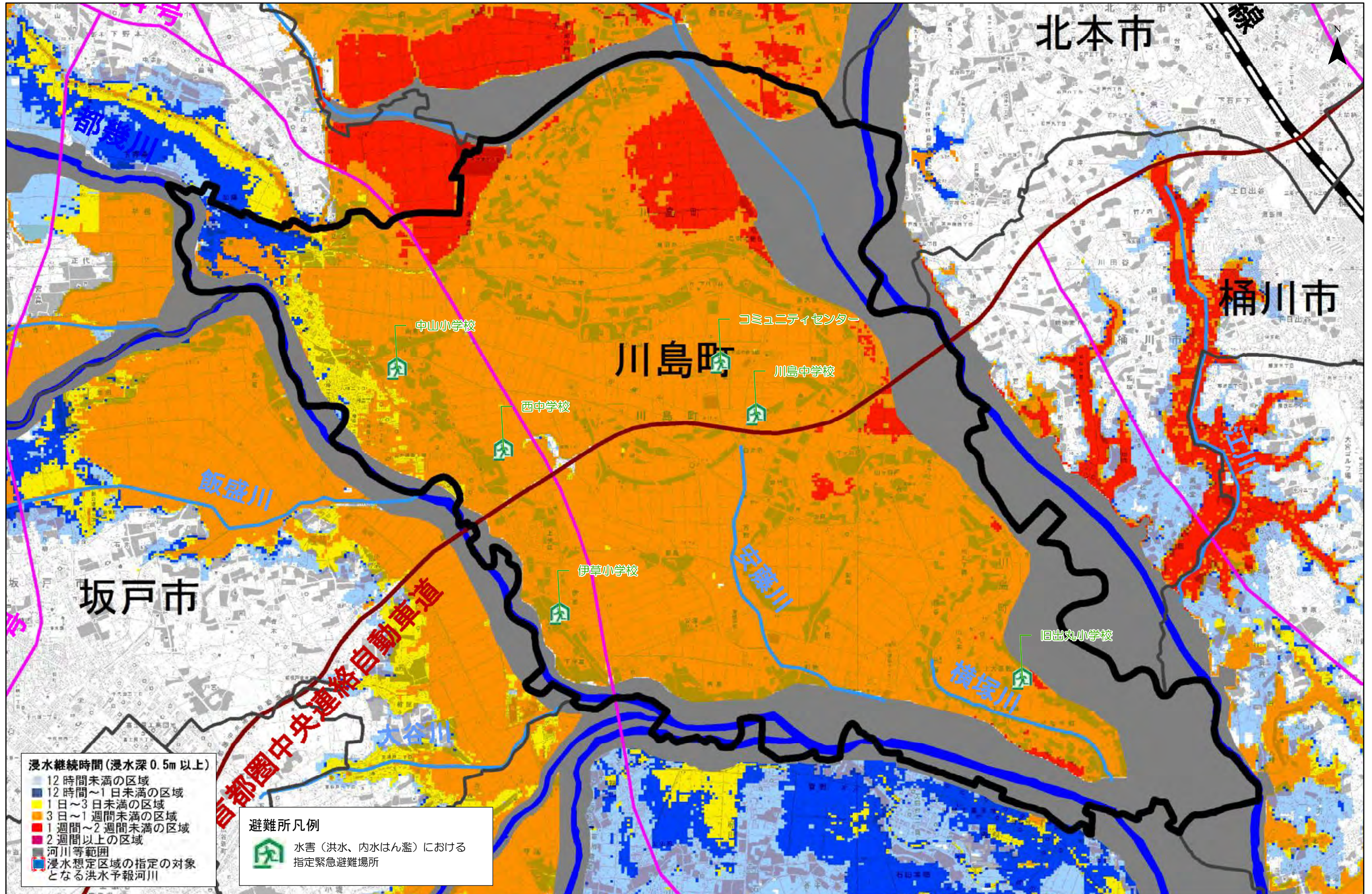
荒川水系荒川及び入間川流域 洪水浸水想定区域図（浸水継続時間）と川島町の避難所
