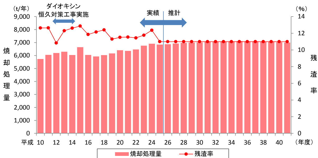
図 2-2-18 焼却処理量の予測結果（現状推移時）
