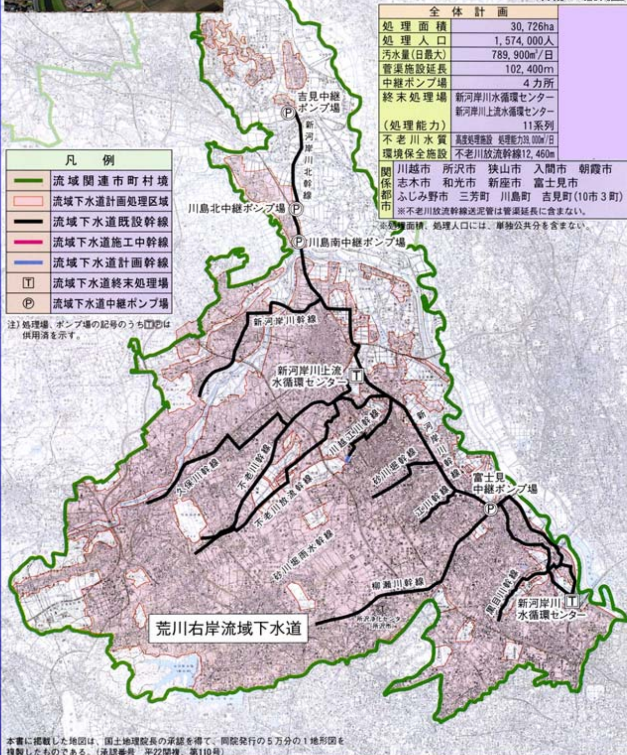
図2-3-2 荒川右岸流域下水道の概要
