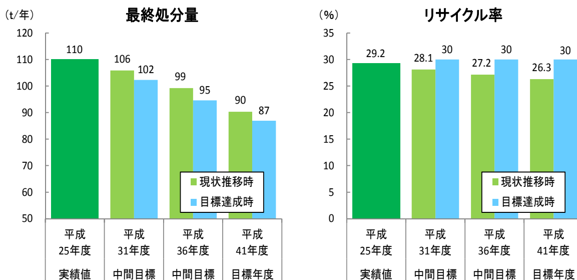
図 2-2-22 現状推移時と目標達成時の最終処分量、リサイクル率
